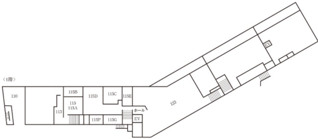
1階平面図
