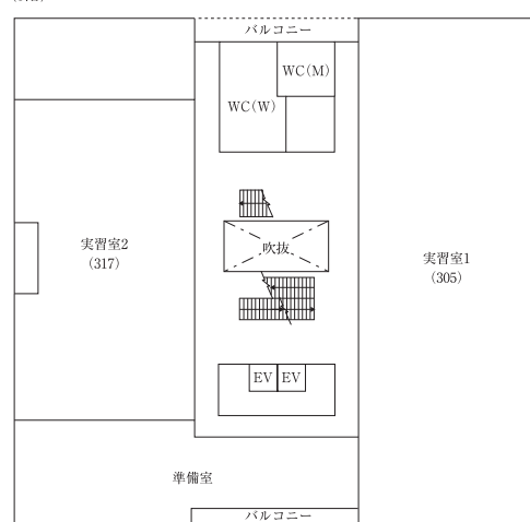
〈3階〉
