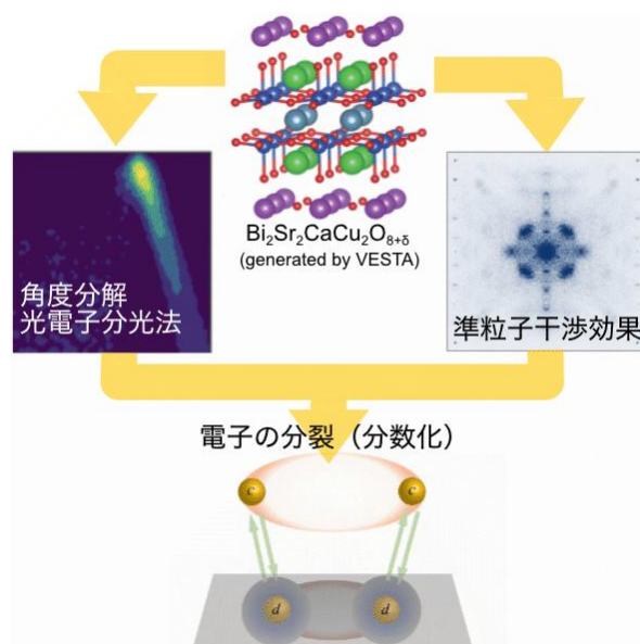
図：本研究の概略。銅酸化物 \text{Bi}_2\text{Sr}_2\text{CaCu}_2\text{O}_{8+\delta} について測定された角度分解光電子分光法及び準粒子干渉効果の実験データを統合解析し、高温超伝導の鍵となる電子の分数化の実験的証拠を得た。
